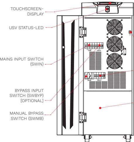
ACTIVE 60 kVA (Vorderseite)
