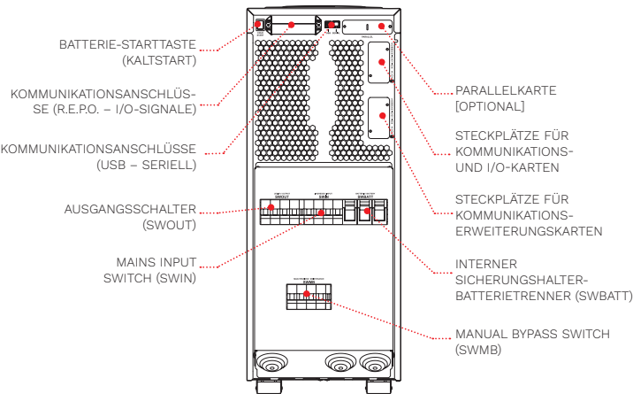
COMPACT 10–20 kVA (Rückseite)
